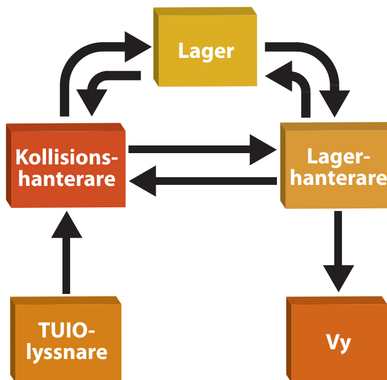
Figur 5.5: Mjukvaruprototypens delar
